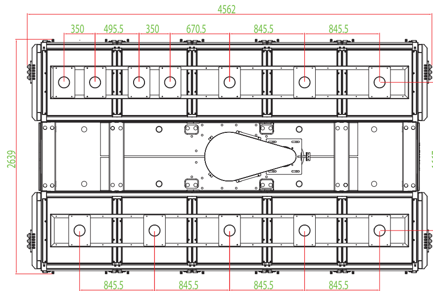
GMJ 10-8
