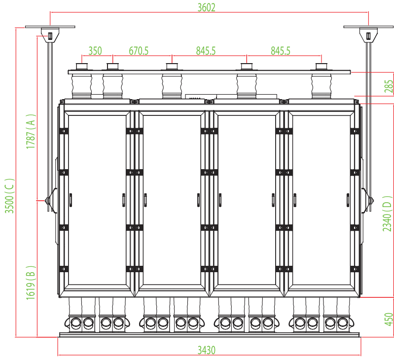
GMJ 8 (30-28-24-20-16)
