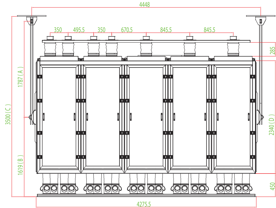
GMJ 10 (30-28-24-20)
