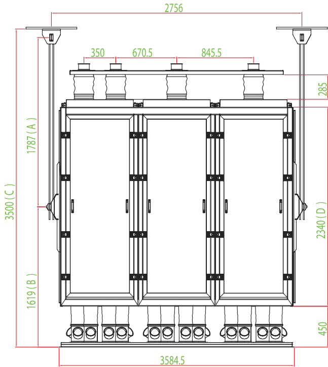
GMJ 6 (30-28-24-20-16)
