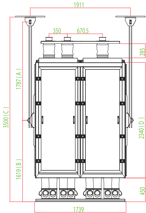
GMJ 4 (30-28-24-20-16)
