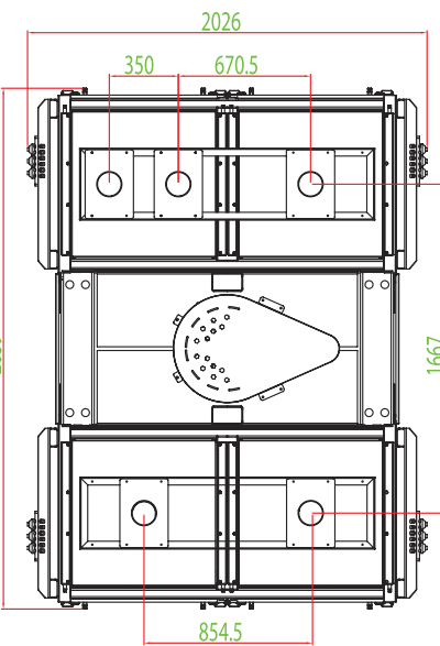
GMJ 6-4
